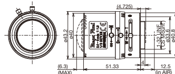
M13VG246
